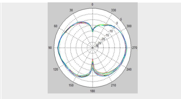
5.8G 垂直面方向图
