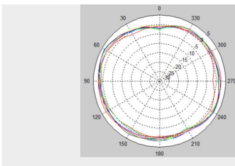
5.8G 水平面方向图
